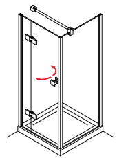
PADEA 230 Pendeltür und Fixteil mit Seitenwand
