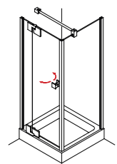
TIBA 230 Pendeltür am Fixteil mit Seitenwand
