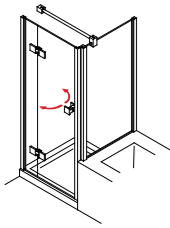
PADEA 231 Pendeltür und Fixteil mit verkürzter Seitenwand
