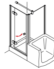
ARANO 231 Drehtür am Fixteil mit verkürzter Seiten- wand
